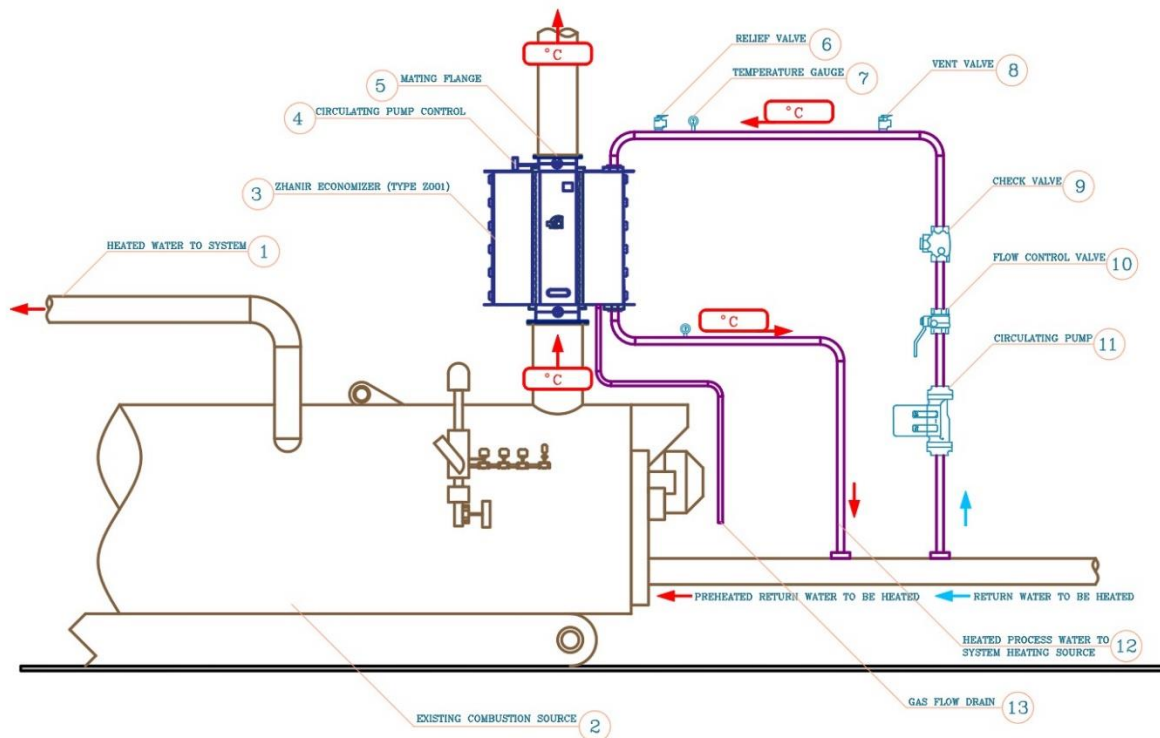
نمونه سیکل پیش گرمایش آب برگشتی به دیگ
