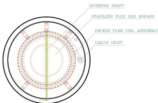
بازیاب حرارتی دیگ آب گرم مدل zhanir 001 - شرکت توانیر-
